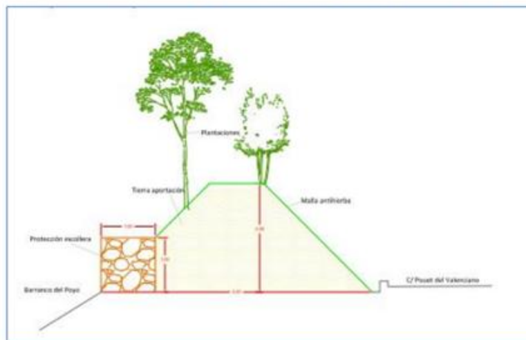
Figura 2. Sección tipo de la mota (Extraída de la documentación aportada)
