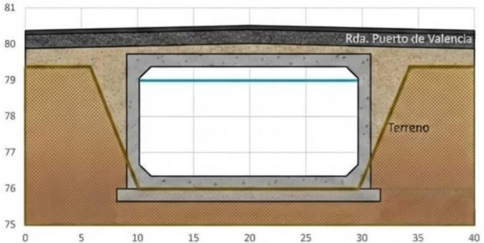
Posible sección de la estructura transversal en la Rda. Puerto de Valencia
