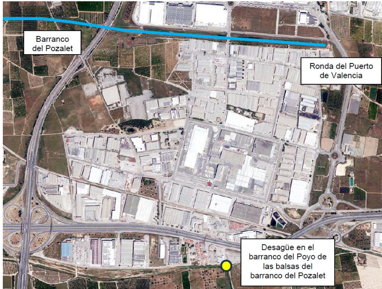
Balsas entre A-7 y ronda del Puerto de València
