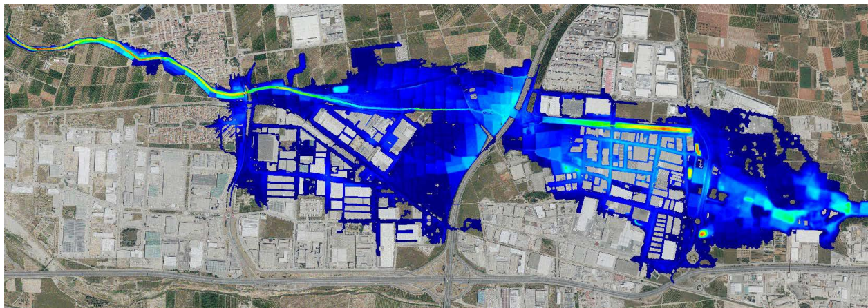
Situación actual con caudales DANA en el barranco de Pozalet
